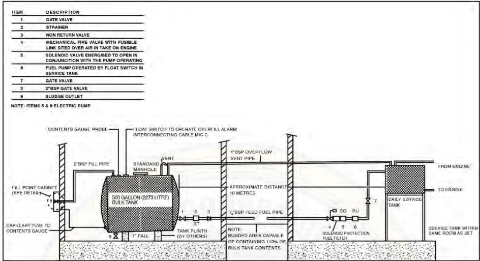
شکل ۴.۳. نقشه نصب پیشنهادی برای مخازن اصلی و روزانه
