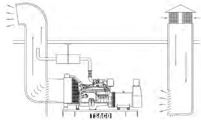
شکل ۳-۵. روش صحیح تهریه هوا
