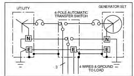
شکل ۱۰،۳ ارتباط ۳ فاز ۳ سیم ۳ قطب وصل شده
