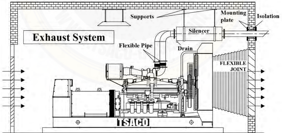
شکل ۵.۱. تیپ عمومی سیستم اگزوز
