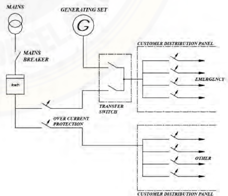
شکل ۹.۱. روش نصب یک سیستم اضطراری رایج
