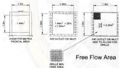
شکل ۳-۴. بازشویی ورودی و خروجی هوا
