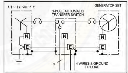
شکل ۱۰،۲ اتصال ۳ فاز ۳ سیم به زمین و اتصال نول به زمین
