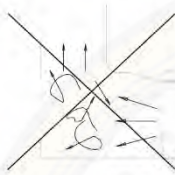
شکل ۳-۳. روش ناصحیح هدایت جریان هوای گرم رادیاتور
