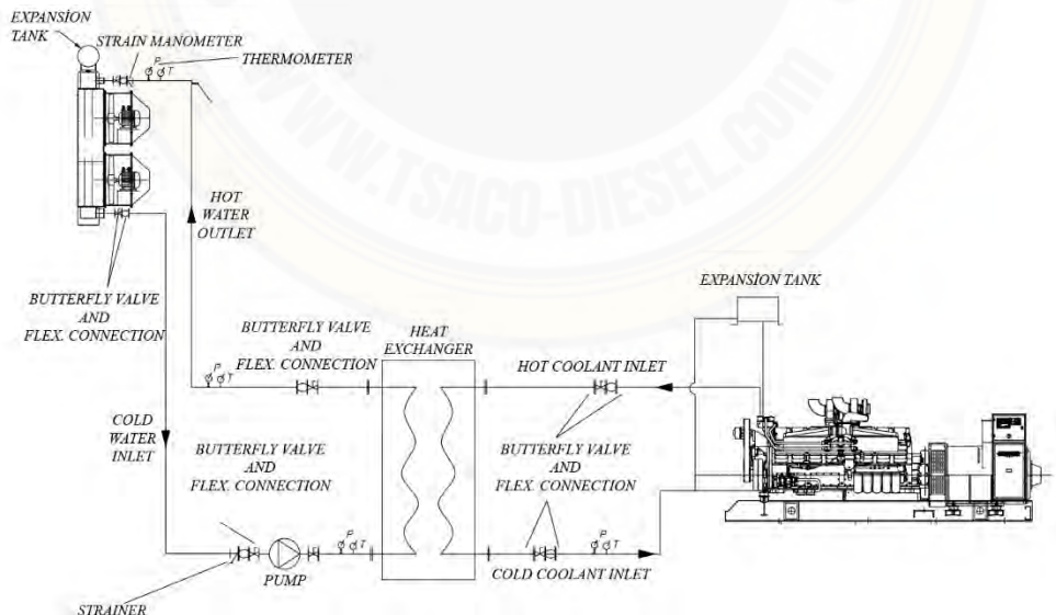
شکل ۶،۳ - سیستم خنک کاری معمول با مبدل حرارتی
