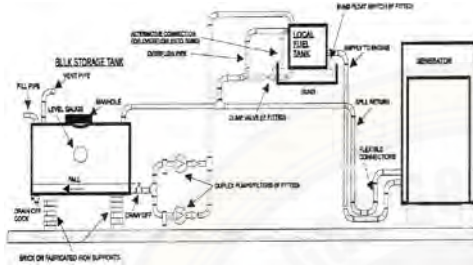
شکل ۴.۱. بدون مخزن سوخت روزانه میانی
