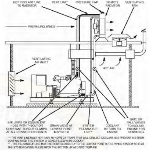
شکل ۶،۲. سیستم خنک کاری با ریموت رادیاتور معمول
