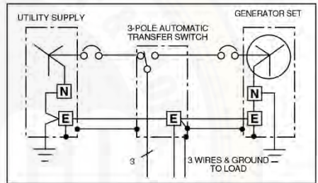
شکل ۱۰،۱ اتصال ۳ فاز ۳ سیم
