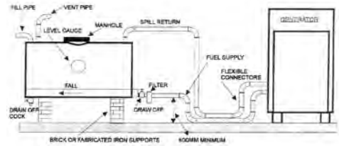
شکل ۴.۲. با مخزن سوخت روزانه میانی
